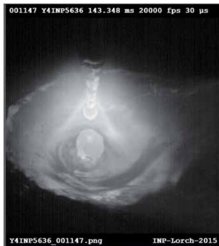
Bild 2: Der Primärtropfen hat sich gelöst und die Sekundärtropfen bilden sich.
