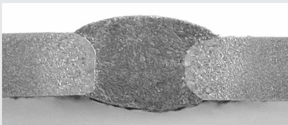
Optimales, leicht überwölbtes Nahtbild ohne Bindefehler – für ein Höchstmaß an Spalttoleranz und Spaltüberbrückung.
