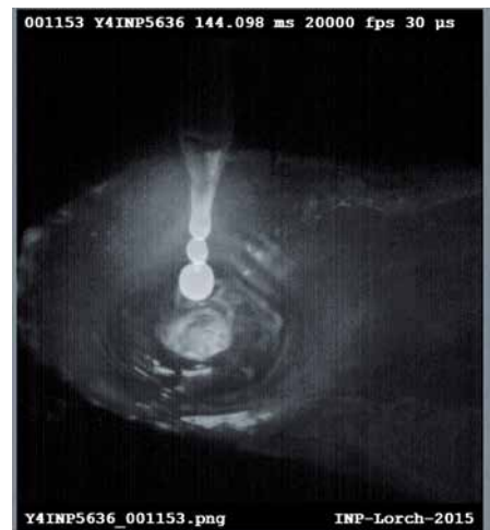
Bild 3: Der Primärtropfen geht ins Schmelzbad über und die Sekundärtropfen lösen sich.
